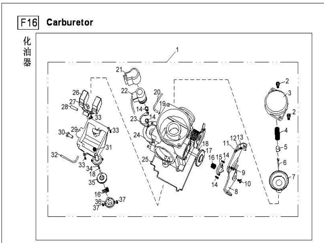
F16 Carburetor
